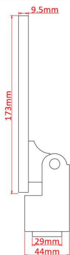
侧面示意图
