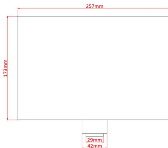
正面示意图
